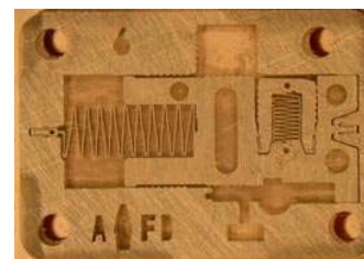
MEMS Layer
